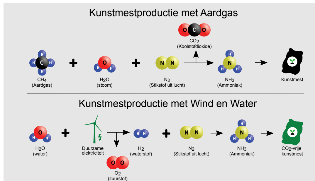
Figuur 9: Kunstmest kan ook gewoon met water, elektrolyse en duurzame elektriciteit gemaakt worden.
