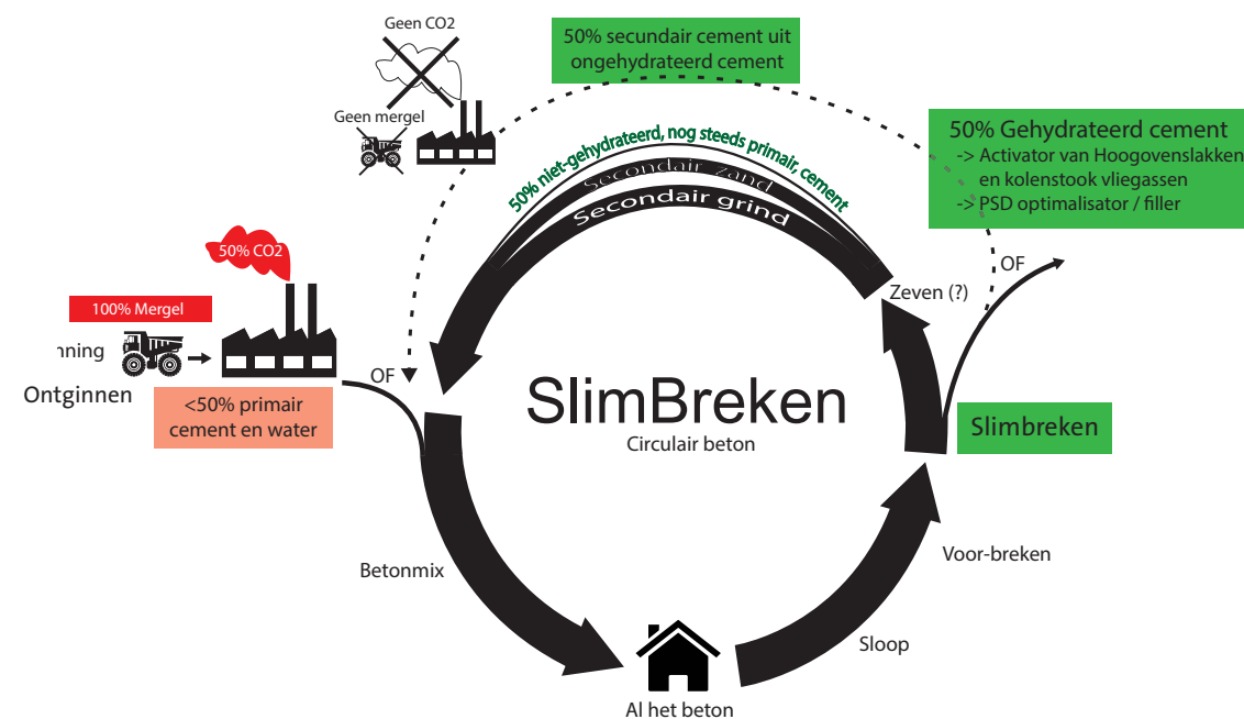
Figuur 11: SlimBreken zorgt voor beton met veel minder \text{CO}_2 -uitstoot.
